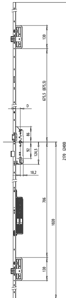
Doornmaat 35 – 45 - 55 – 65mm Lengte 2170 of 2400 – V24x3mm
