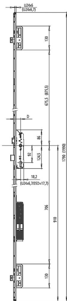
Doornmaat 35 – 40 – 45mm Lengte 1790 of 1990 - U24x6mm
